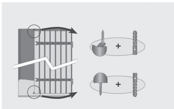
Butées haute et basse pour poste bois
