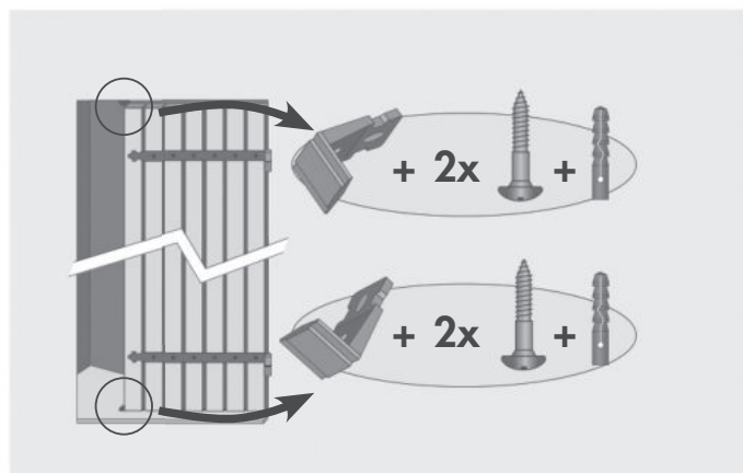
Butées haute et basse pour porte PVC et aluminium
