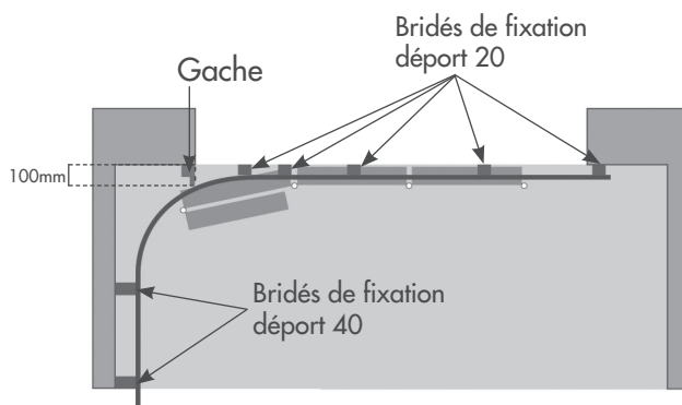
Vue de dessus de la porte montée
