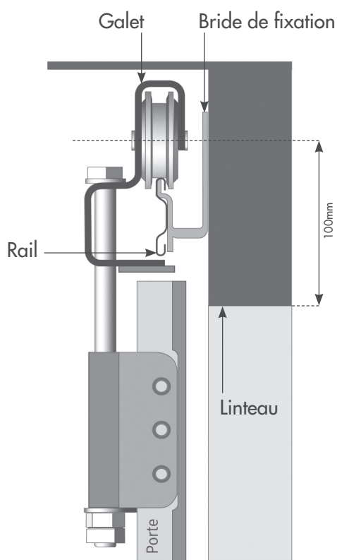
Fonctionnement du guidage haut (rails, galets, panneaux)
