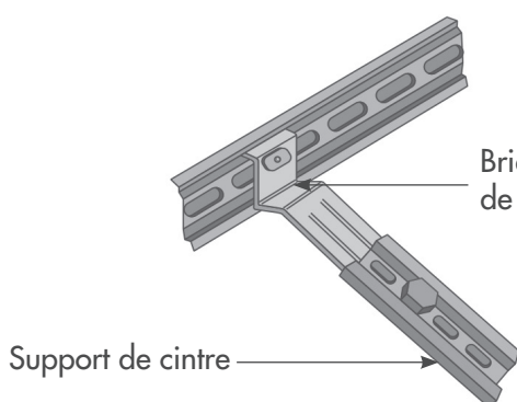
Principe d'assemblage du support de cintre et du raccord de rail
