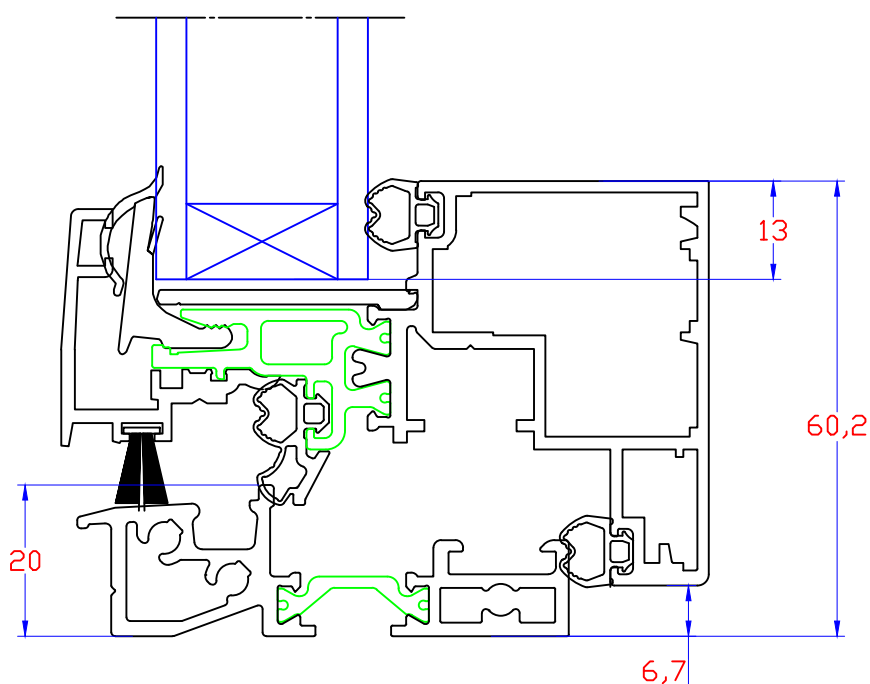
Seuil avec Ouvrant Caché
