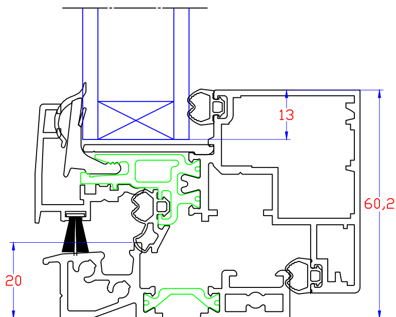
Vue en coupe verticale traverse basse avec seuil
