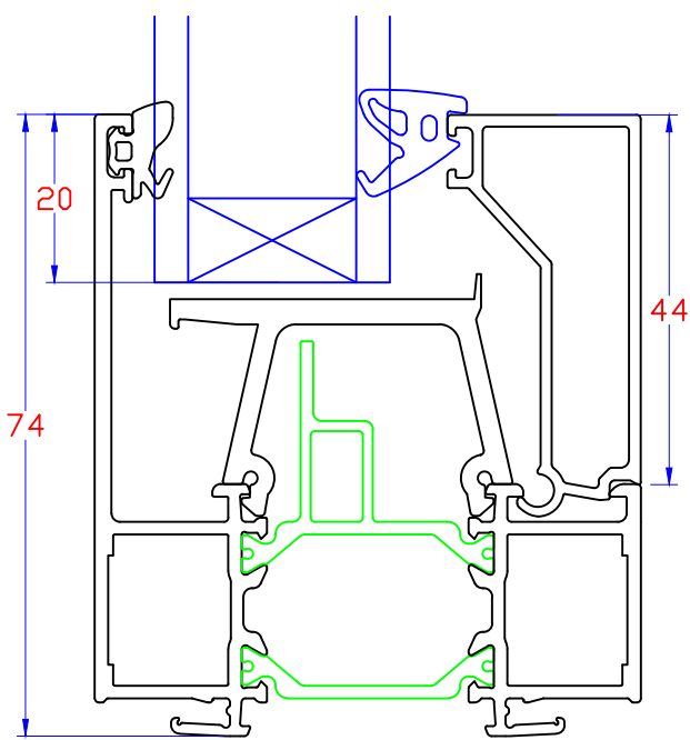
Vue en coupe verticale sur fixe
