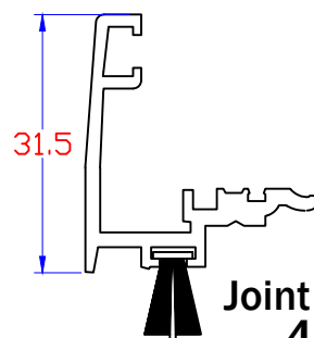
Rejet d'eau pour seuil Ouvrant Caché Y3710007
