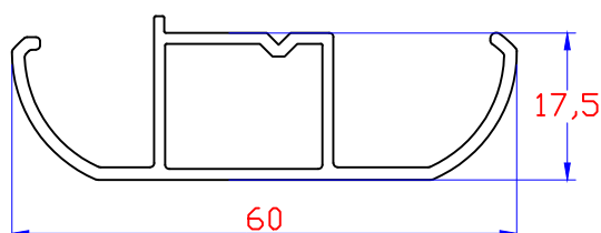
Battement Intérieur OC Galbé W3090108
