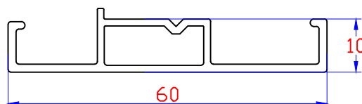
Battement Intérieur OC Carré Y3710004
