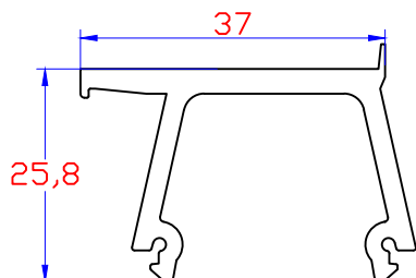
Support de Cale pour vitrage fixe W8020003
