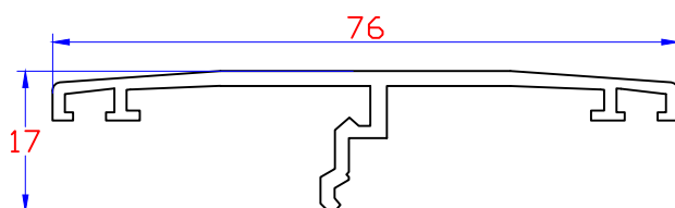
Battement Extérieur Y3710012 (pré-percé)
