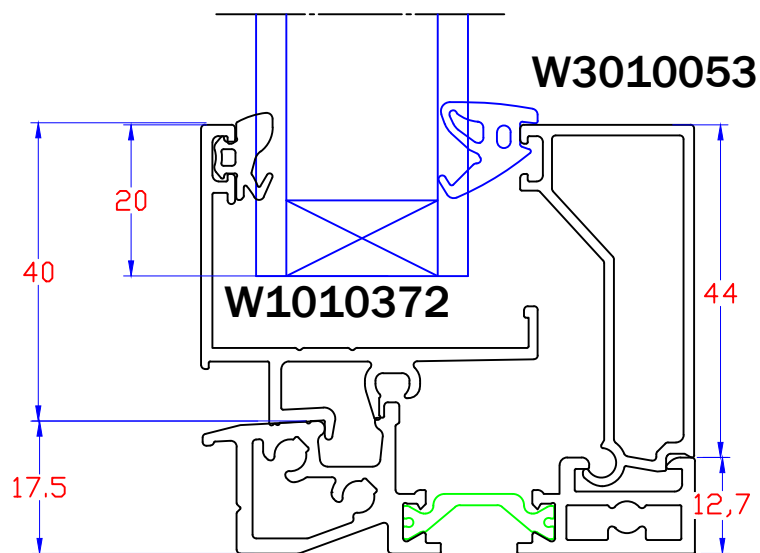
Feuillure rapportée + pareclose
