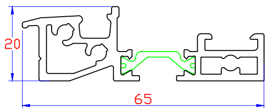
Seuil avec Ouvrant Caché
