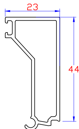
Pareclose pour fixe W3010053
