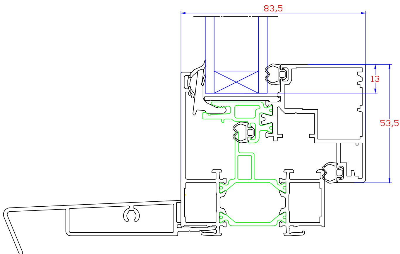
Vue en coupe verticale traverse basse avec appui
