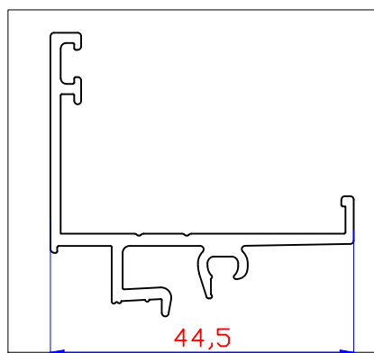
Feuillure rapportée W1010372
