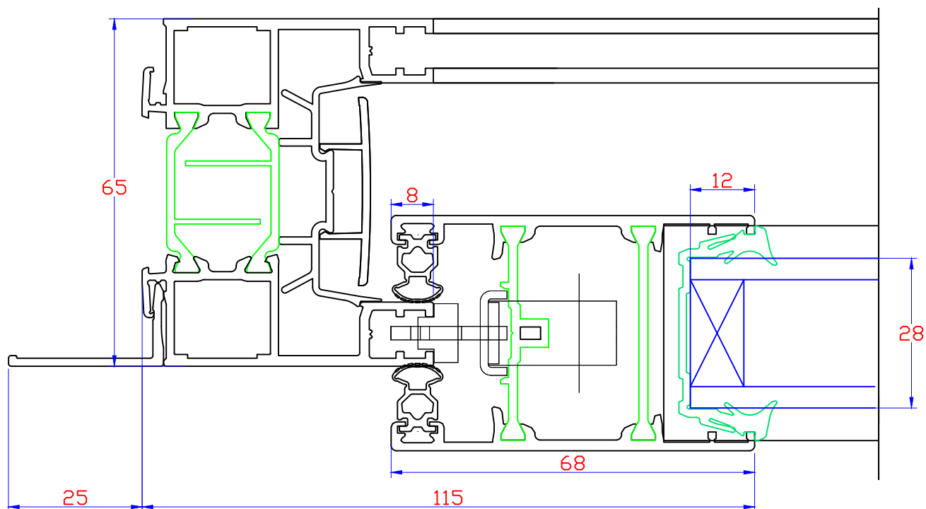
Vue en coupe sur montant central
