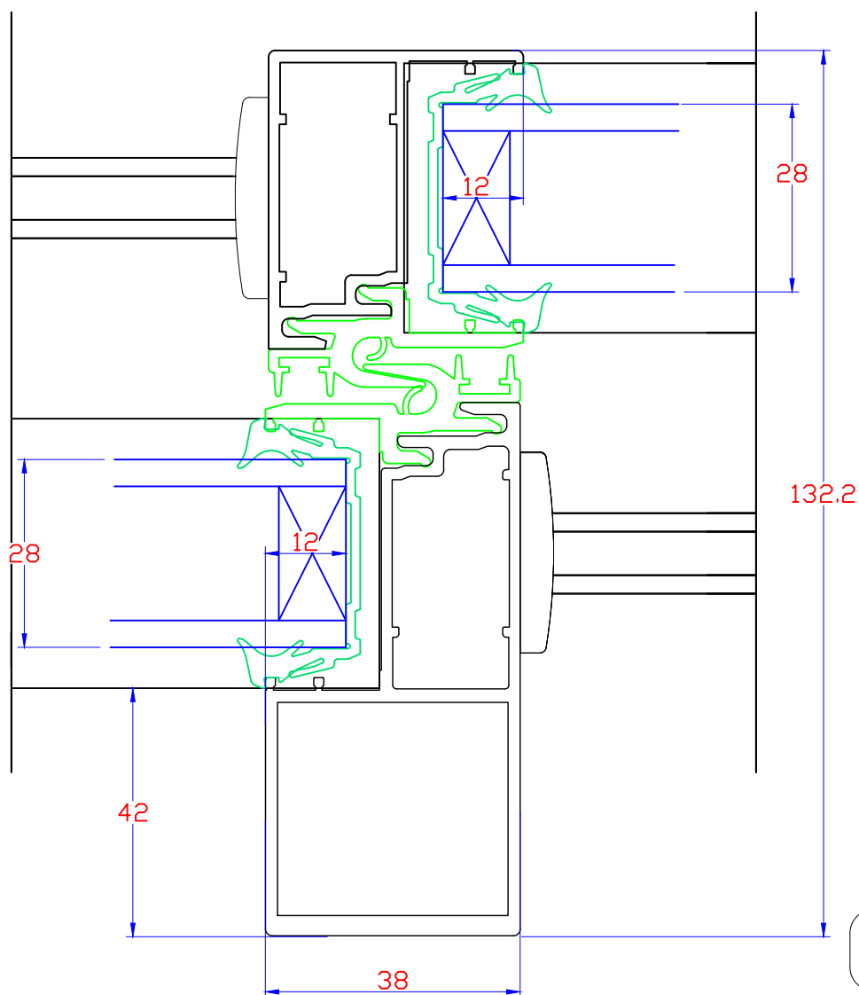
Vue en coupe sur montant central
