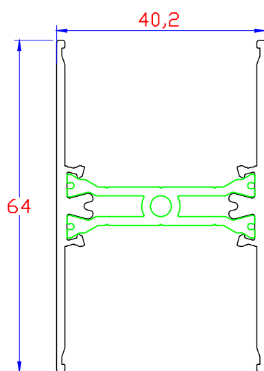
Traverse Intermédiaire W1041275
