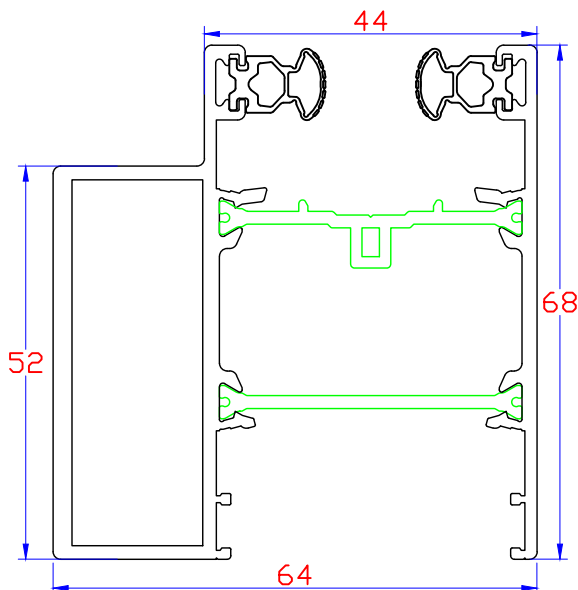
Montant Latéral Forte Inertie W1041272
