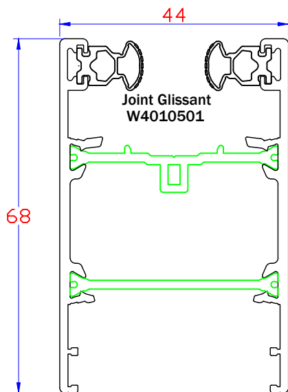
Ouvrants Montant Latéral W1041270
