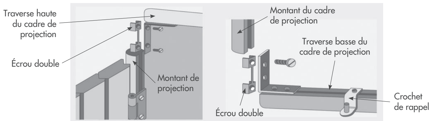
Principe d'assemblage du cadre de projection
