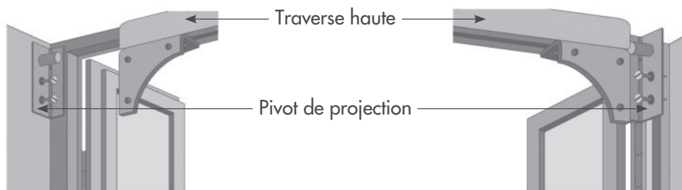
Assemblage de la traverse haute avec les pivots de projection
