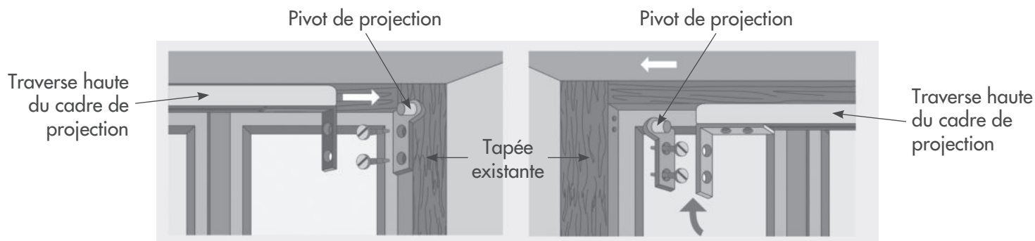
Assemblage de la traverse haute avec les pivots de projection
