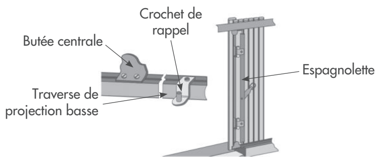
Butées haute et basse
