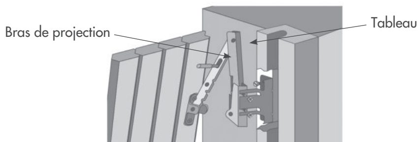
Principe de Fonctionnement du cadre de projection
