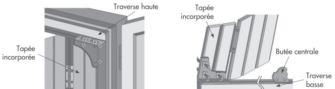
Principe d'assemblage de la tapée incorporée sur le cadre de projection
