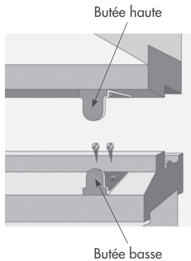
Butées haute et basse
