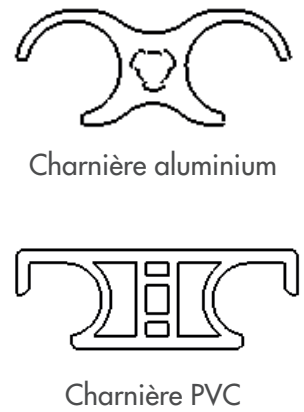
Vue en coupe - Charnière
